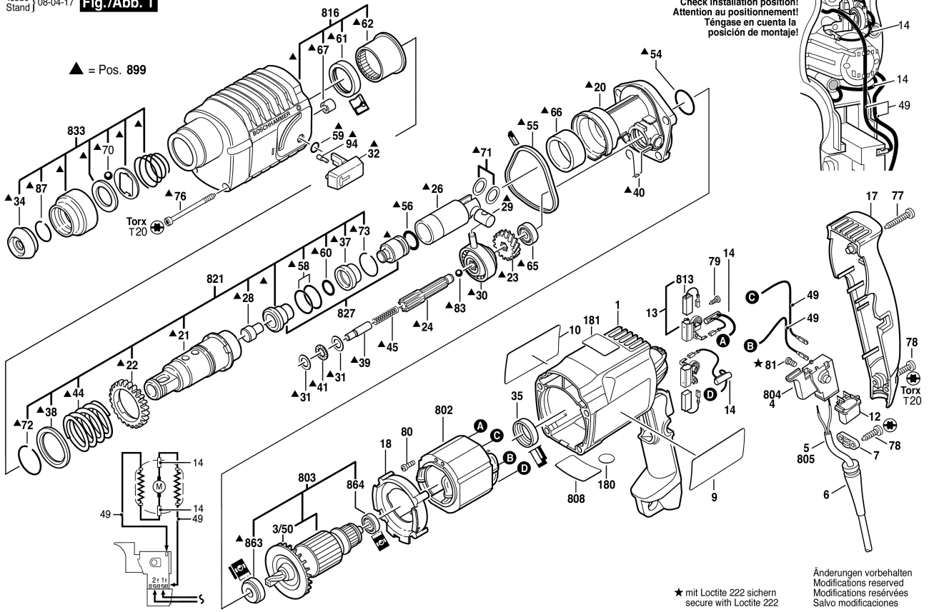
Fig./Abb. 1
