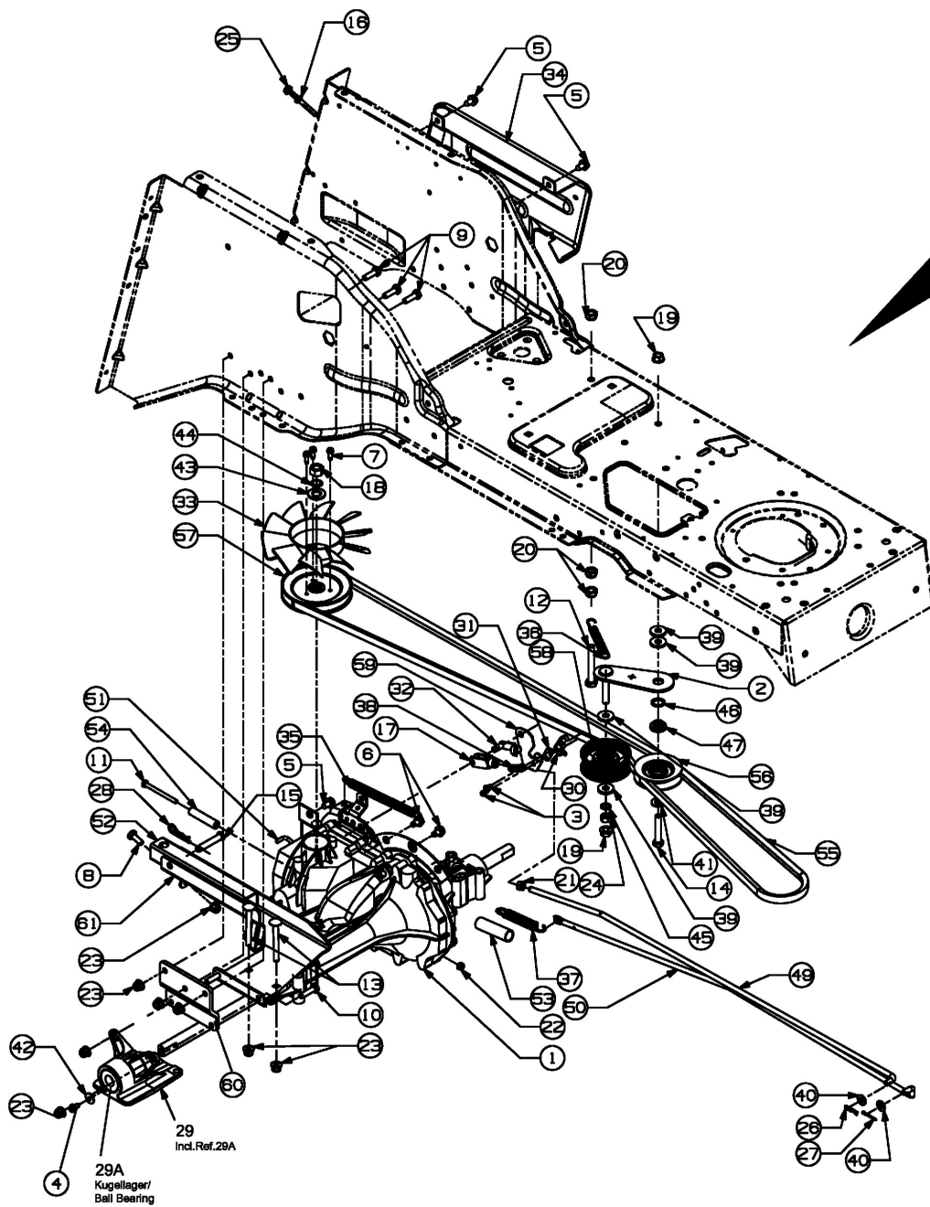
Seitenansicht / Side view A
