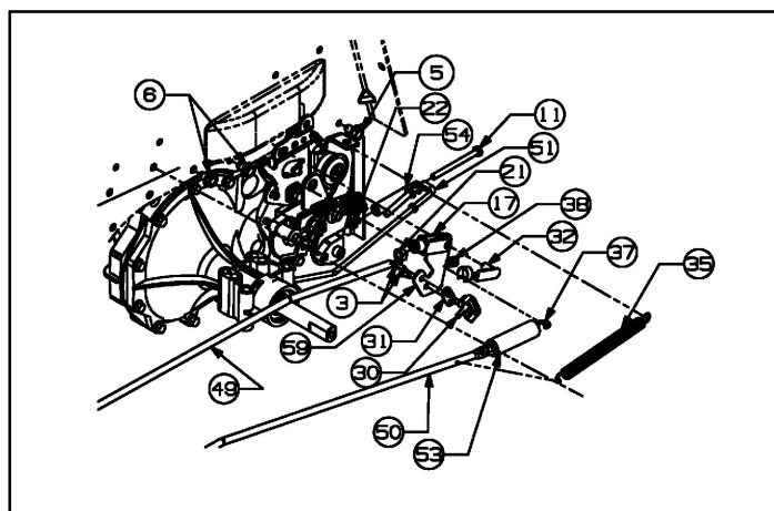
Seitenansicht / Side view A
