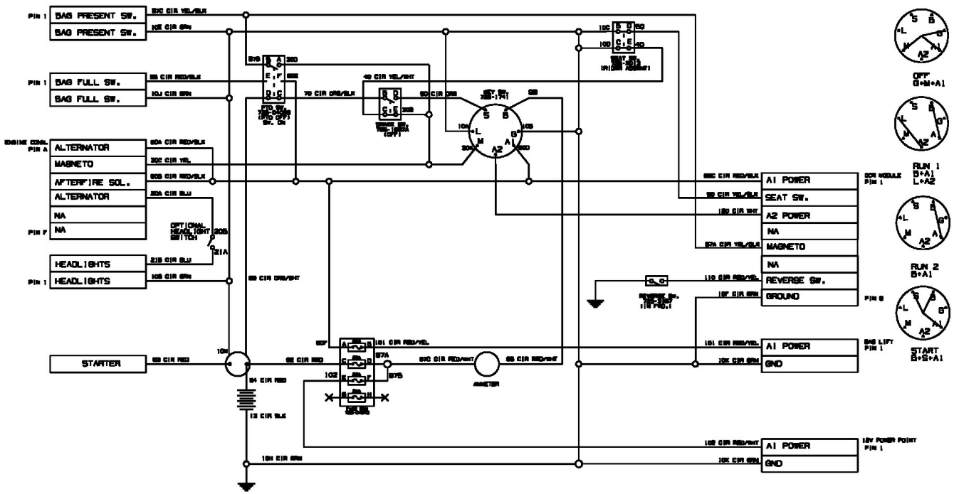
Schaltplan / Diagram
